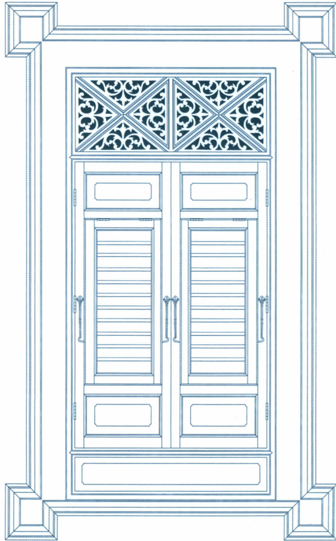
ลายไม้ฉลุช่องแสงเหนือหน้าต่างบานเปิดแบบกระทุ้งติดบานเกล็ด
