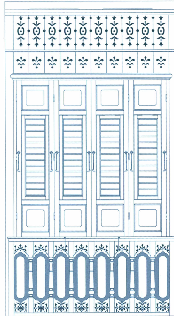
ลายไม้ฉลุประดับช่องแสงเหนือหน้าต่างและพนักลูกกรงใต้หน้าต่าง บริเวณมุขห้าเหลี่ยม
