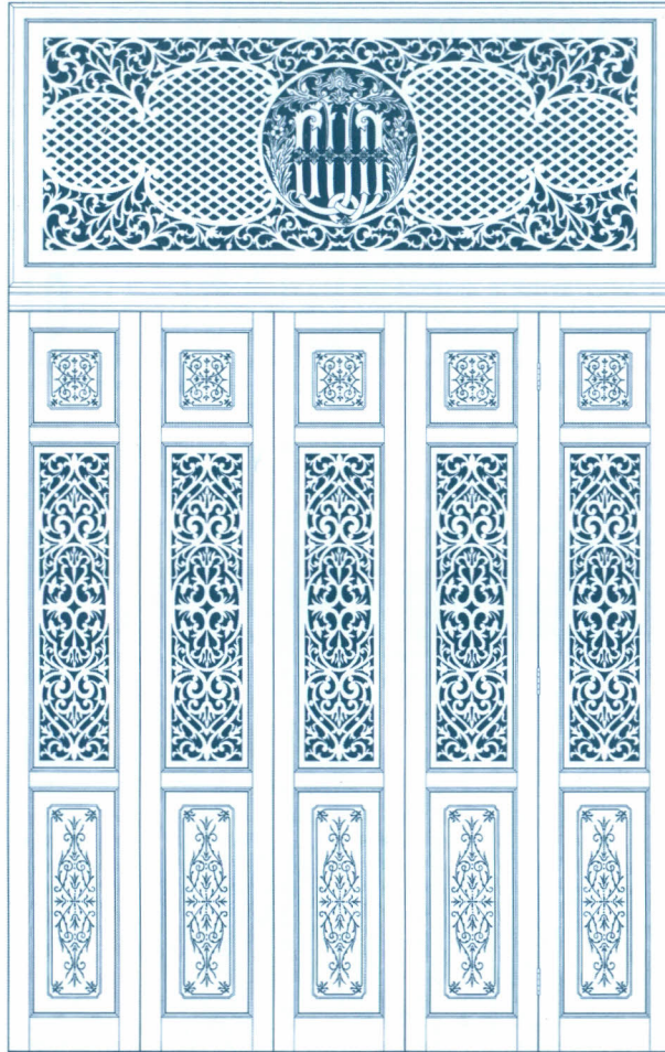
ลายไม้ฉลุประดับประตูบานเพิ่ม (แบบที่ ๑)
